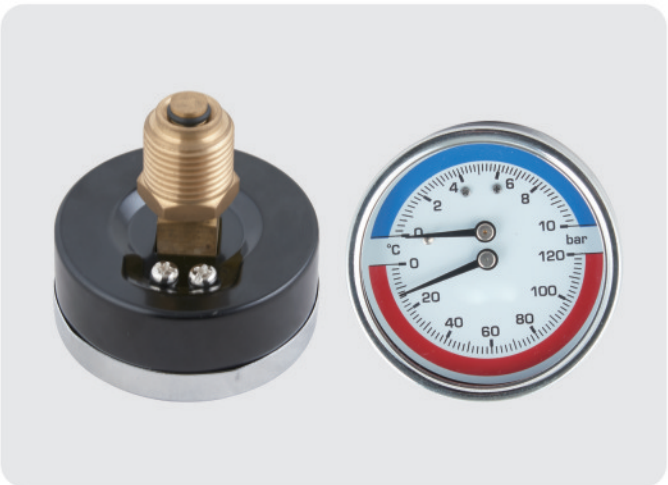
温度压力表 Temperature gauge
